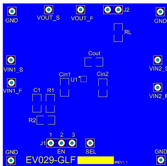
Fig 2. Bottom Layer
