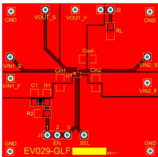
Fig 1. Top Layer
